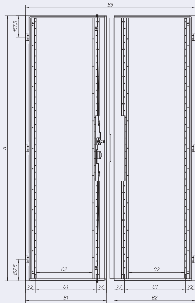
Ajtók XVTL-D...
