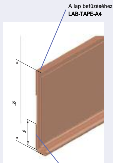
Öntapadó csík
