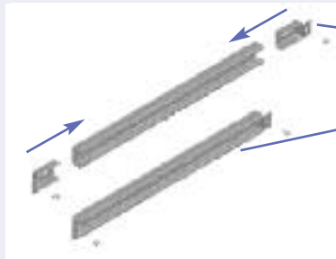
BPZ-KAS kábelrögzítő-sín, leszerelve
