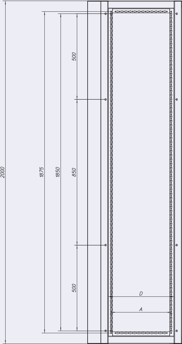
Sarokmezők XVTL-CF/S-...
