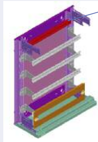
BPZ-KAS kábelrögzítő-sín, összeszerelve, az alapteretbe szereléshez kész
