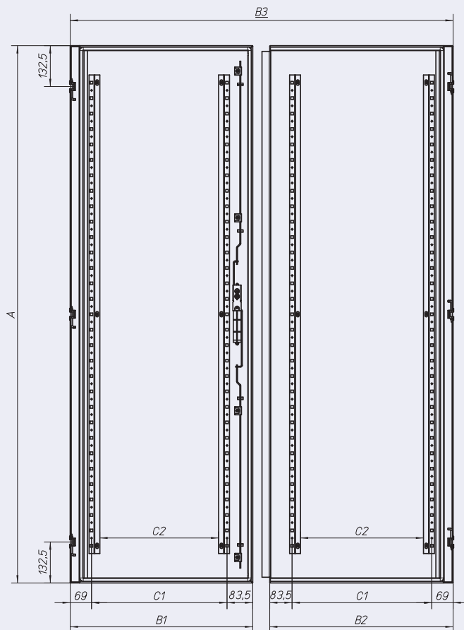
Ajtók XSDMC...
