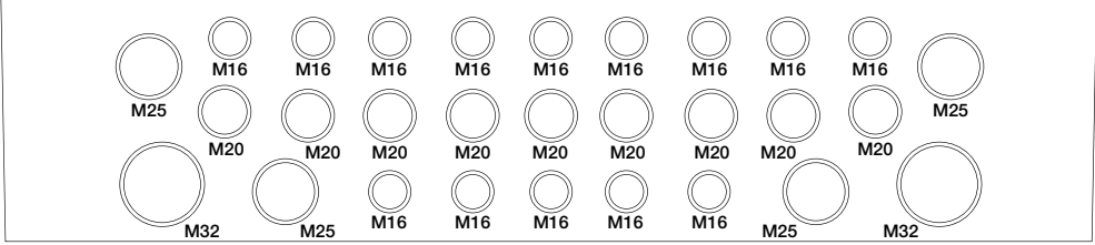
18 modul - alsó és felső
