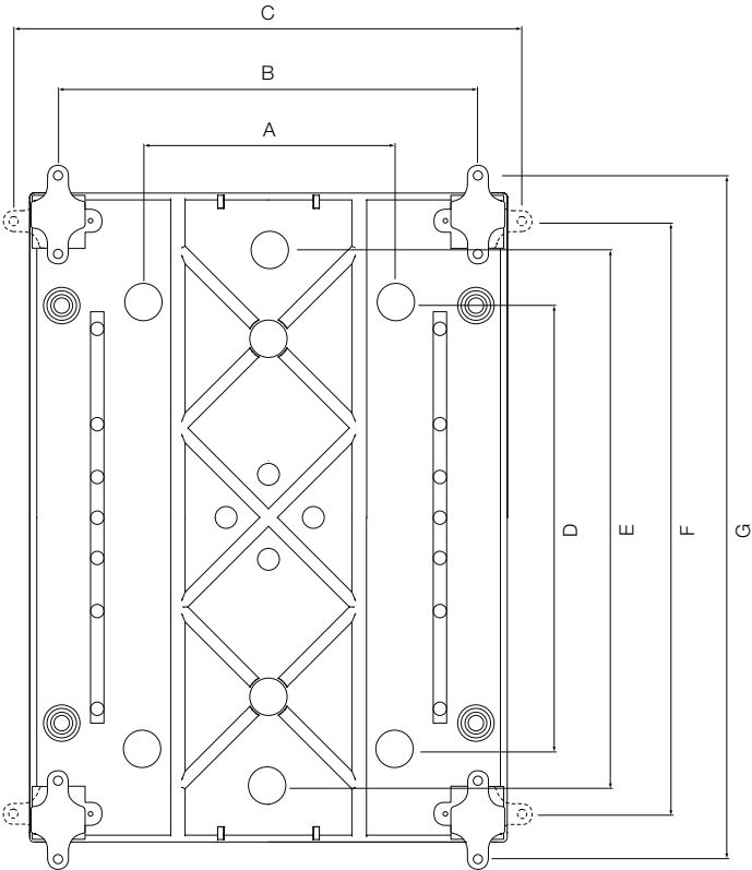
Fúrósablon
