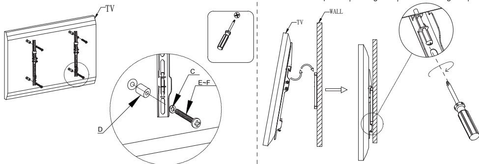
3. A tv rögzítése a fali lemezhez és a biztonsági csavar beillesztése / Atașarea televizorului la placa de perete și adăugarea șurubului de siguranță.
