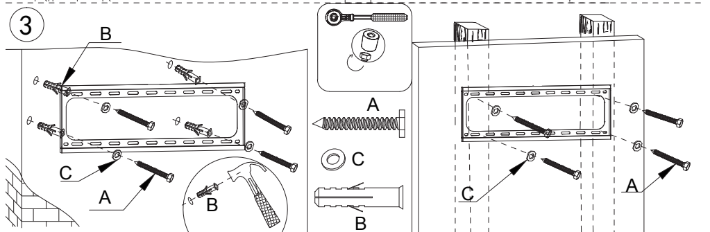
2. Tv-konzolok rögzítése lapos háttapú televízióhoz / Montarea suporturilor tv pe un televizor cu spate plat
